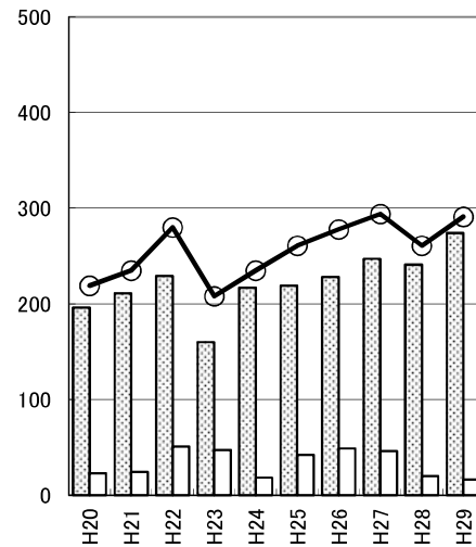
⑧送風機
