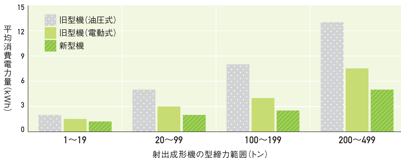
射出成形機の型締力区分別の平均消費電力量
